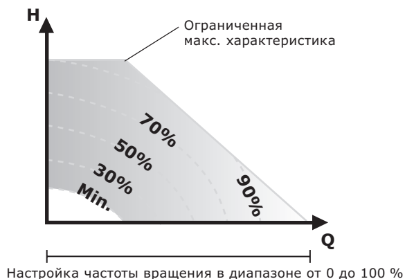
Рис. 58 Ограничения по мощности и давлению, влияющие на максимальную характеристику
