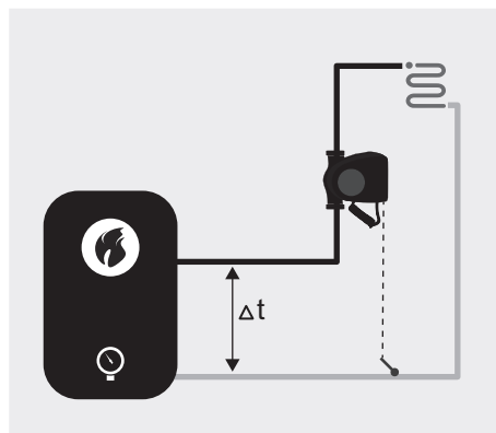
Рис. 56 Перепад температур
