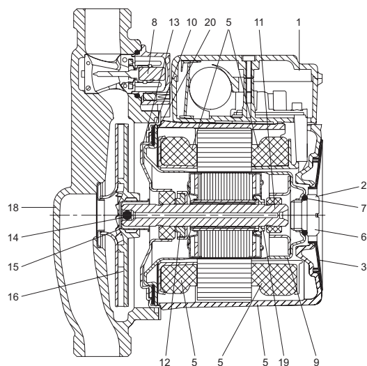
Рис. 62 Разрез насосов PROMO 15-9A, PROMO 15-12A
