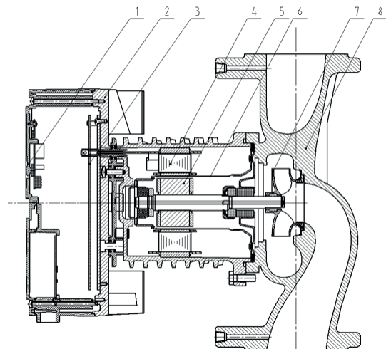
Рис. 59 Автоматический насос MEGA S
