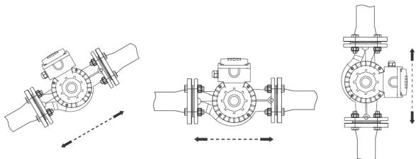
Рис. 60 Варианты монтажа
